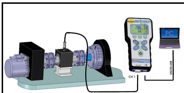
Sistema di misura su banco prova con controllo diretto della COPPIA e della VELOCITÀ tramite ENCODER interno al torsiometro RT2
